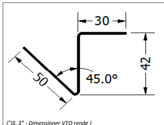
("ill. 3" - Dimensioner VTO rende)
