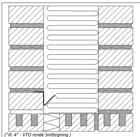
("ill. 4" - VTO rende Snittegning)
