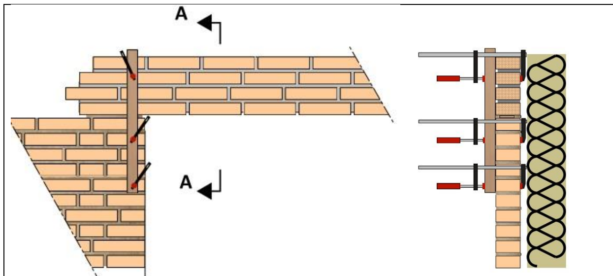
Fig. 4: Eksempel: Fastholdelse mod væltning af prefabrikeret bjælke
