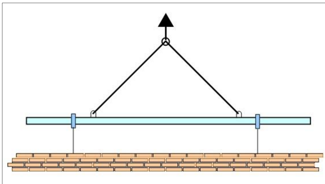
Figur 2: Korrekt løft med åg.
